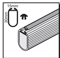
AMS 1702 drażek aluminiowy z uszczelką długość 3m aluminium bar with washer 3m
