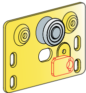
Posizione di aggancio ante Door hookup position Position du crochet du volet Anklinkenstellung der Tür Posición de enganche de la puerta
