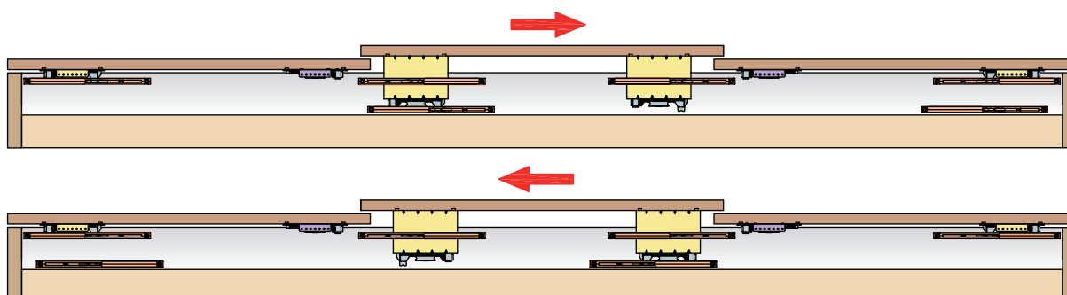
Armadio a 3 ante con 6 fermi ammortizzati in apertura e in chiusura Wardrobe with 3 doors, 6 soft closing for opening and closing
